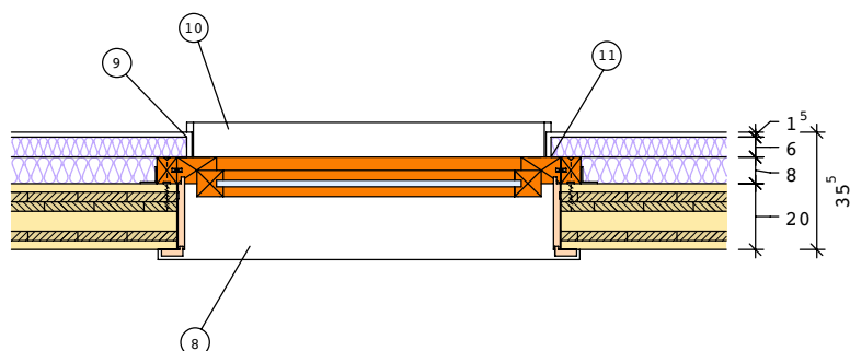
Horizontální řez
