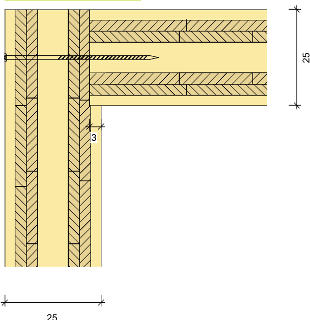
UZAVŘENÉ NAPOJENÍ
