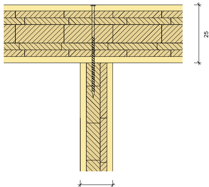
PROVEDENÍ TUPÉ
