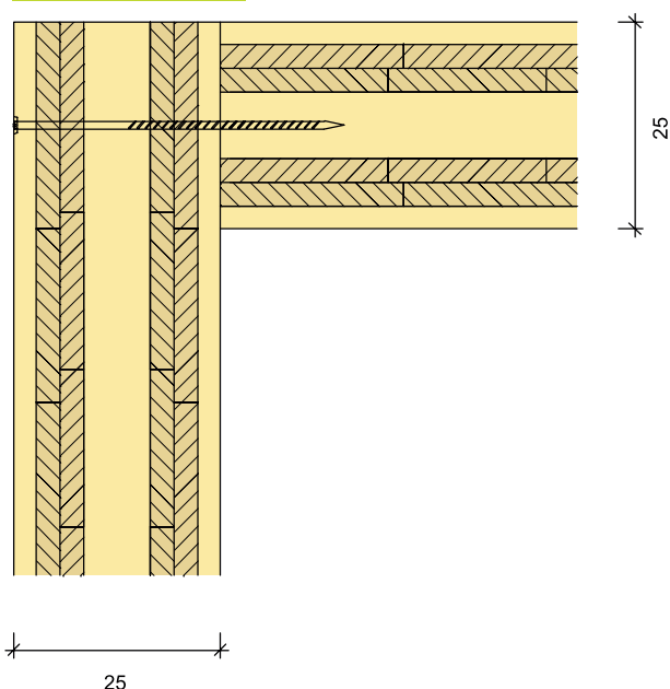
PROVEDENÍ TUPÉ
